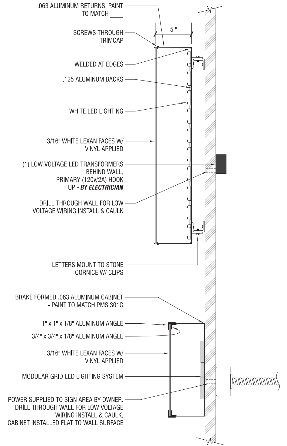
SECTION SCALE: 1 1/2" = 1'-0"
