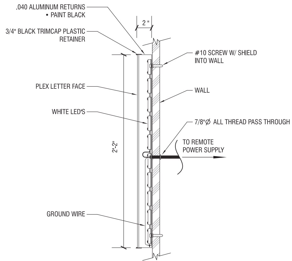
SECTION A SCALE: 1 1/2" = 1'-0"
